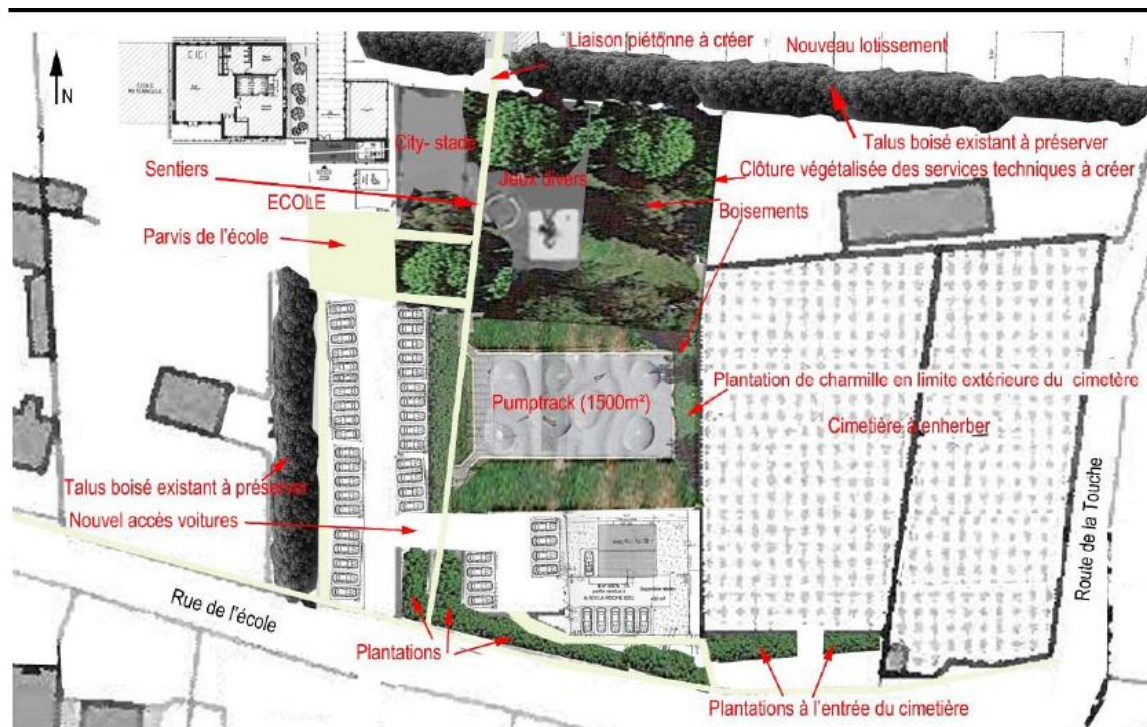
Propositions d'un schéma d'implantation d'un Pumptrack sur une surface d'environ 1500m 2
